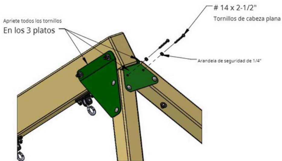
DETALLE A
