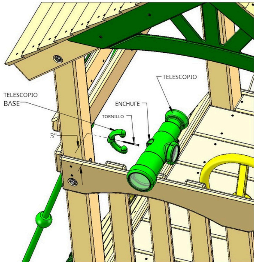
DETALLE A
