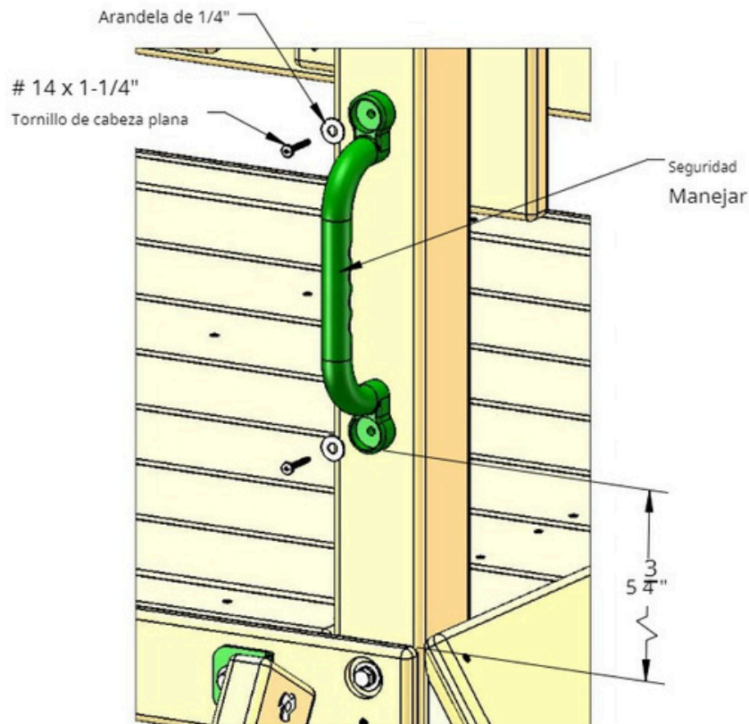
DETALLE A
