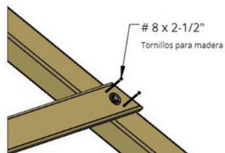
DETALLE B
