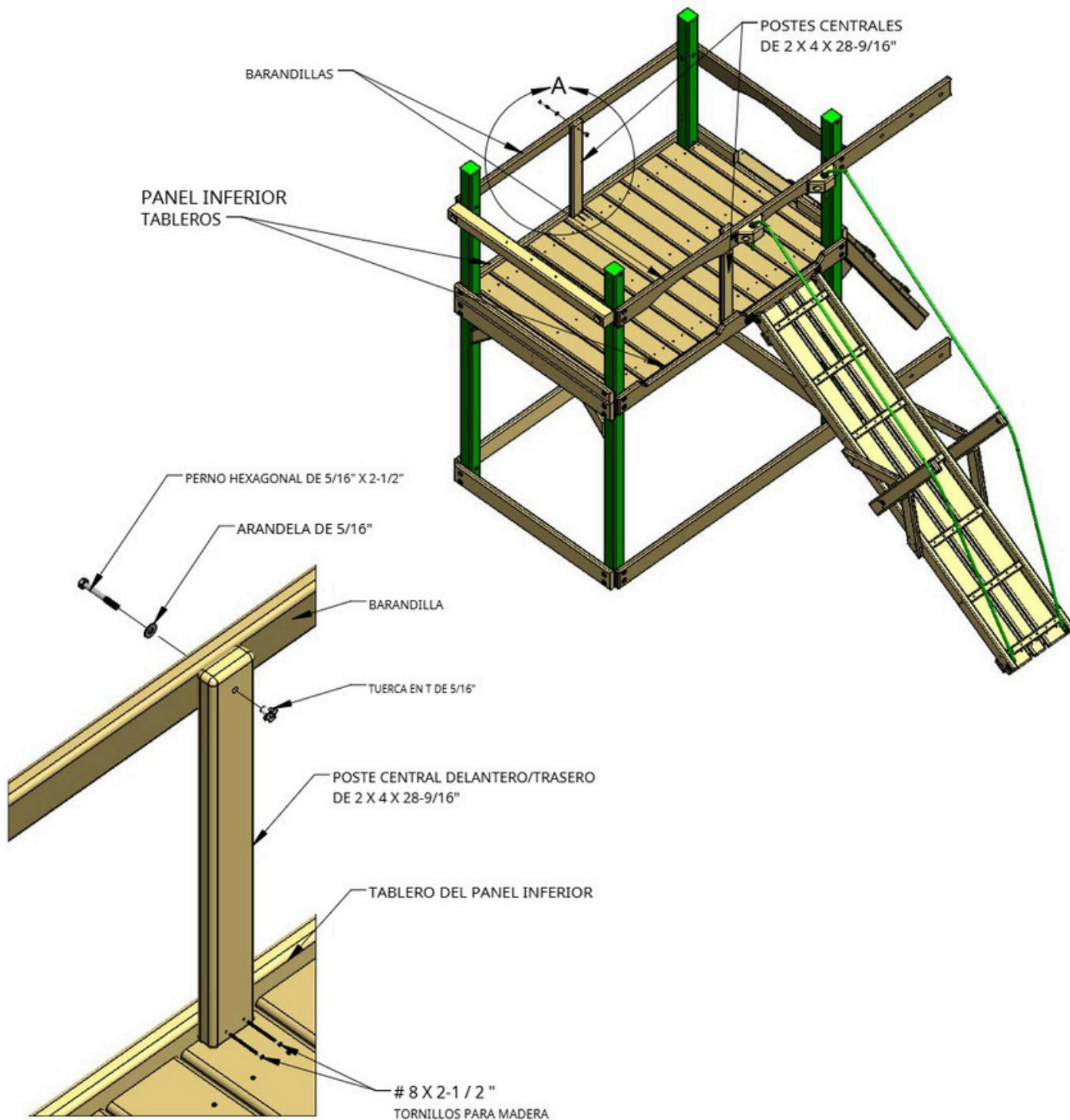
DETALLE A ESCALA 1 : 8
