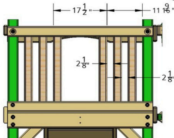
PANEL DE VIGA COLUMPIO SLEN DIMENSIONES (VISTA DESDE EXTERIOR EL ESCENARIO DE JUEGO.)
